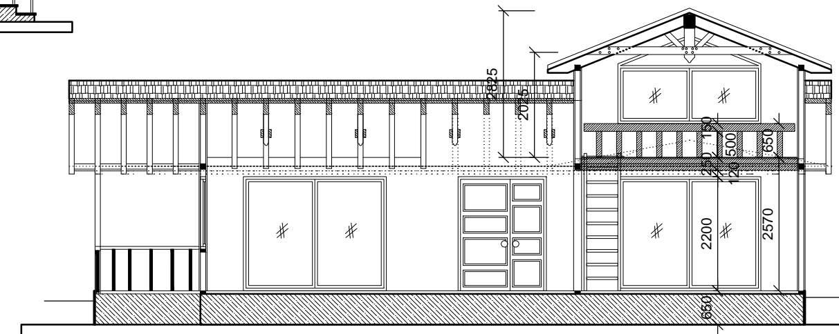
SNID A2-A2
