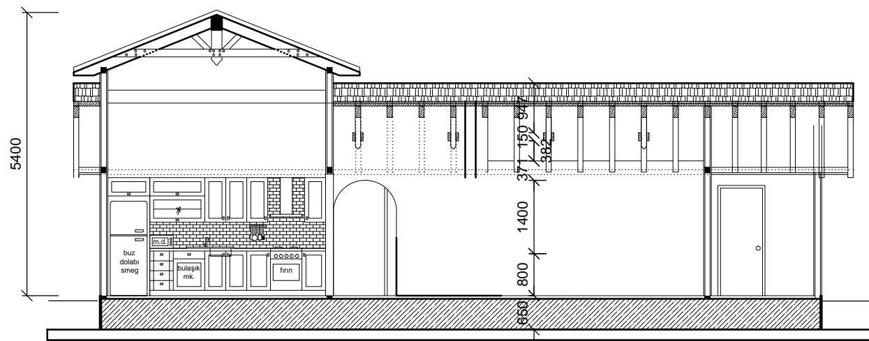
SNID A1-A1
