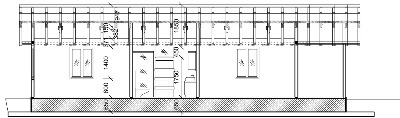
SNID A-A
